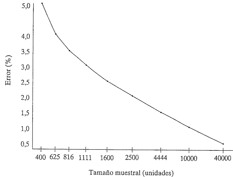
Figura 5.1. Representación gráfica de la relación entre las variables error y tamaño muestral para P = Q = .50 y nivel de confianza del 95,5%.
